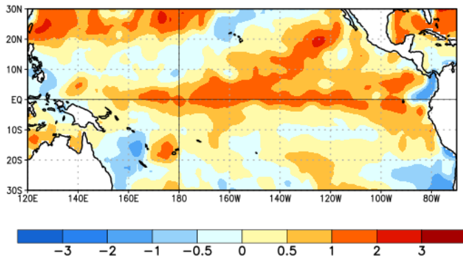
SST Anomalies (°C) 06 MAR 2019
